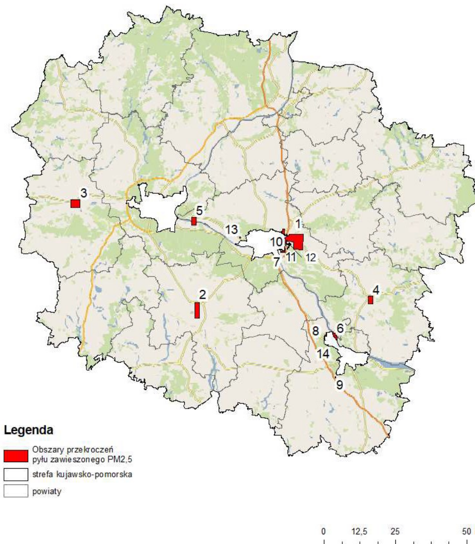
Rysunek nr 4.1.2-2 Obszary przekroczeń średniodobowego poziomu dopuszczalnego pyłu zawieszonego PM 2,5 na terenie strefy kujawsko-pomorskiej w 2021 roku.
